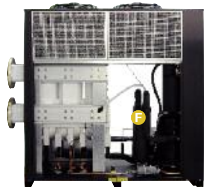
großvolumiger Flüssigkeitsabscheider
