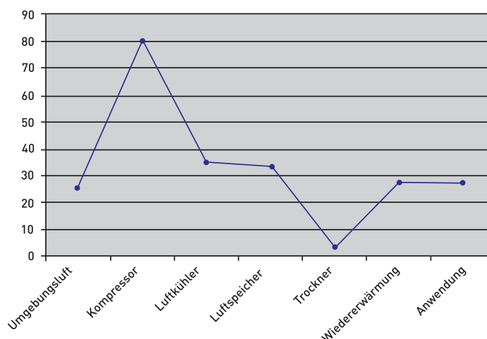
Typische Temperaturen in einem "normalen" Druckluftsystem
